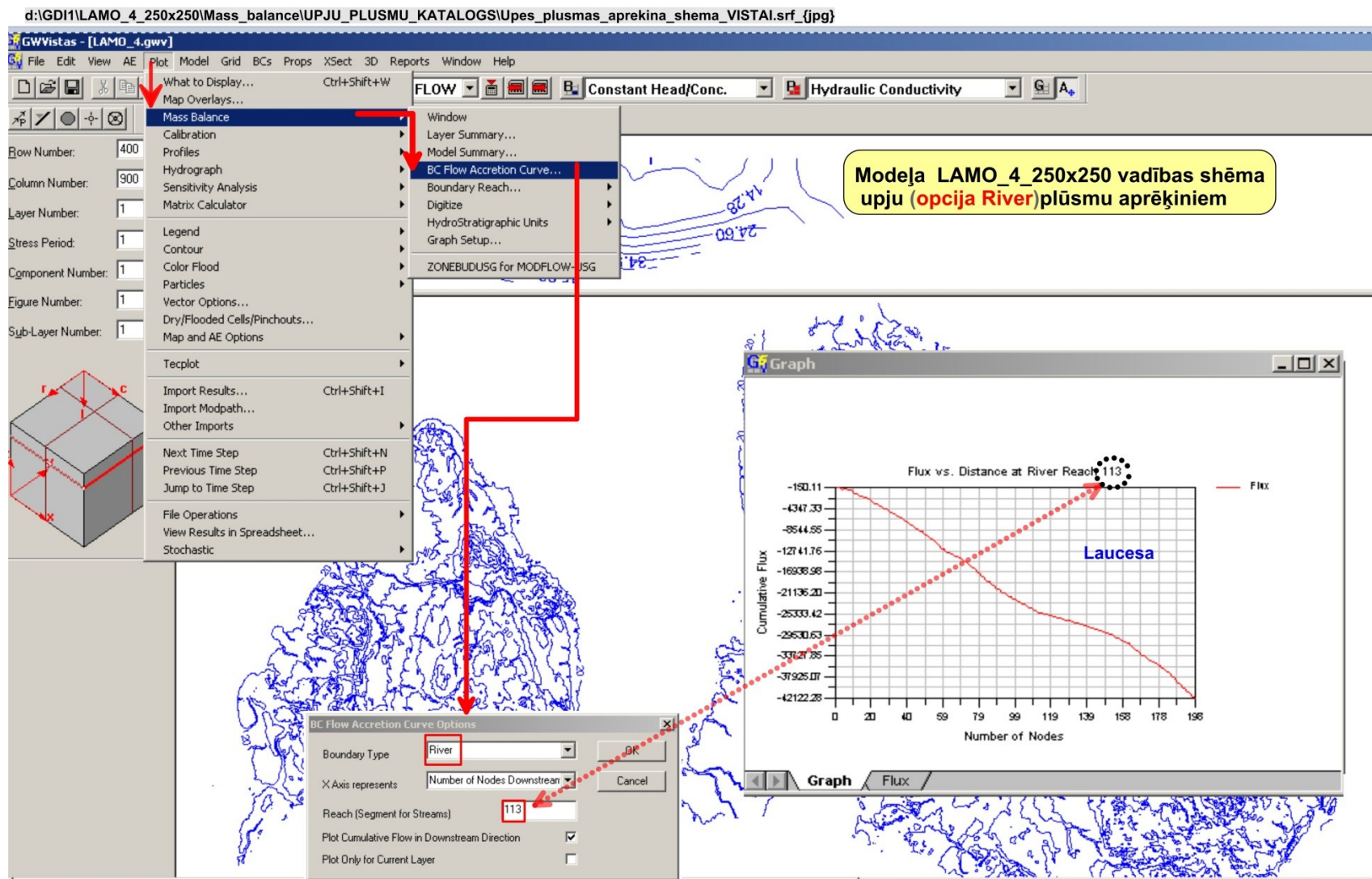
1.att. Upes pazemes pietece plūsmas aprēķina shēma
