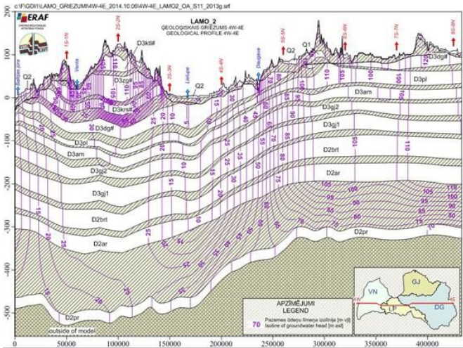
7. att. Ģeoloģiskais griezum 4W-4E LAMO2 versija
