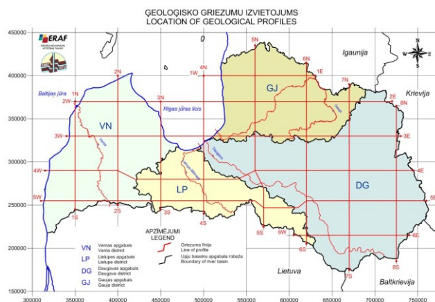
6. att. Latvijas upju lielbaseinu un reģionālo ģeoloģisko griezumņu izvietojums
