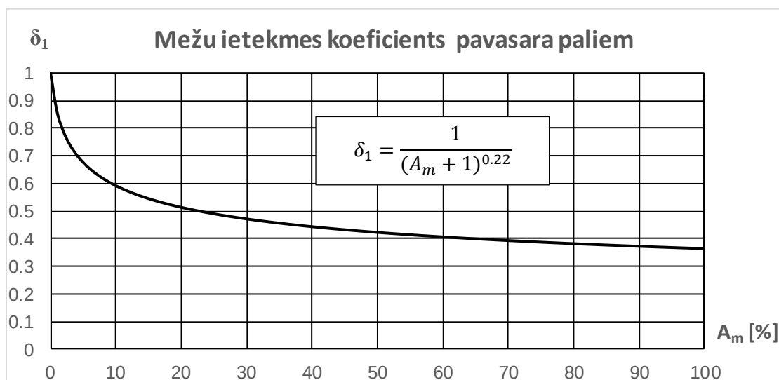
3.4a. att. Pavasara palu aprēķiniem izmantoto parametru grafiki kā laukuma A funkcijas: Pp \text{ [m}^3/\text{s]} , ja A < 25 \text{ km}^2 Pp \text{ [m}^3/\text{s]} , ja A < 2 \text{ km}^2 ; mežu ietekmes koeficients \delta_1
