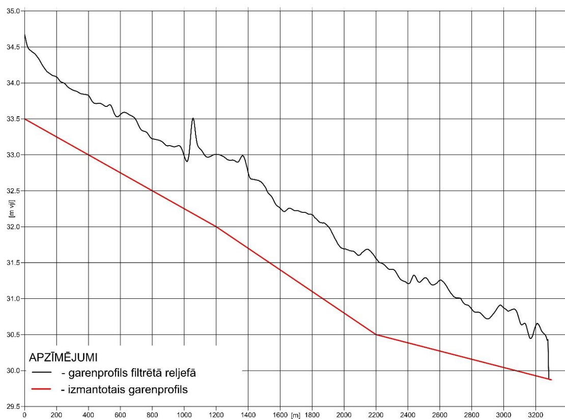
2.9a. att. Saulītes grāvja (2300) ūdens līmeņa profils
