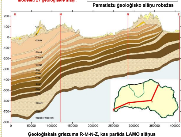
Ģeoloģiskais griezum R-M-N-Z, kas parāda LAMO slāņus
